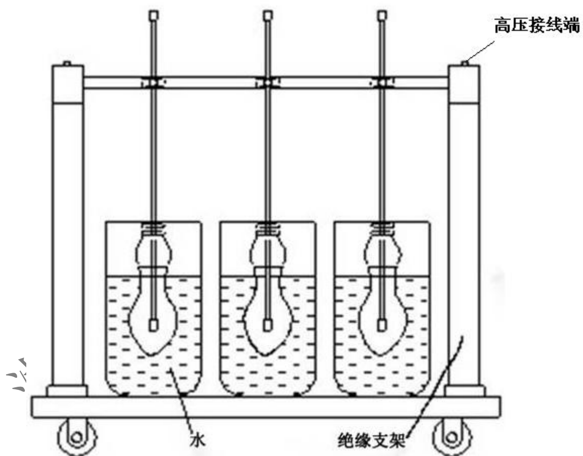
图 3-2 绝缘靴（手套）试验台（侧面图）
