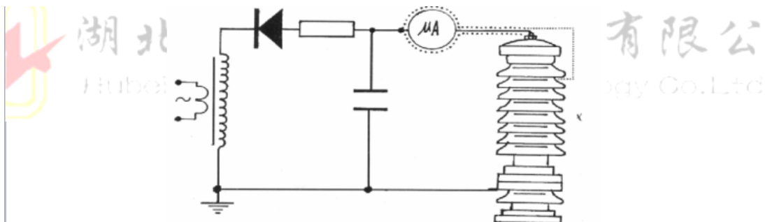
图 7b 排除试品 C_X 表面影响接线图
